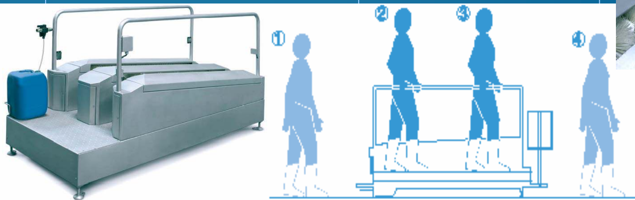
# 12480 station bedoeld als permanent doorloopstation, aanwezigheid wordt geregistreerd d.m.v. foto-cel detectie. Het station is een 2-richtingen wasstation en tevens uit te voeren met ingangs-controlevoorziening met hand-desinfectie.
